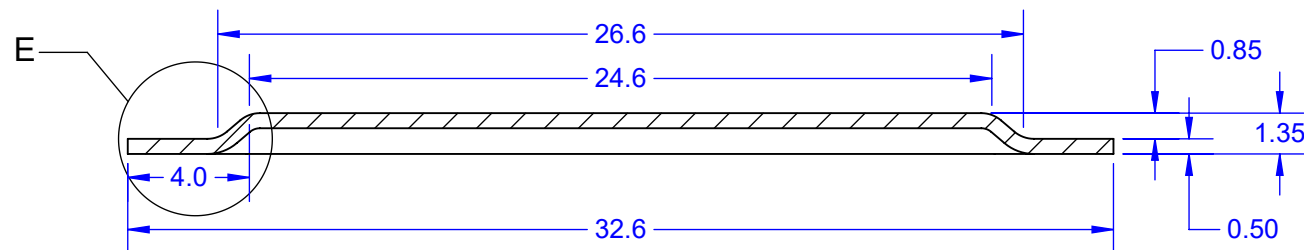
SECTION B-B SCALE 4 : 1
